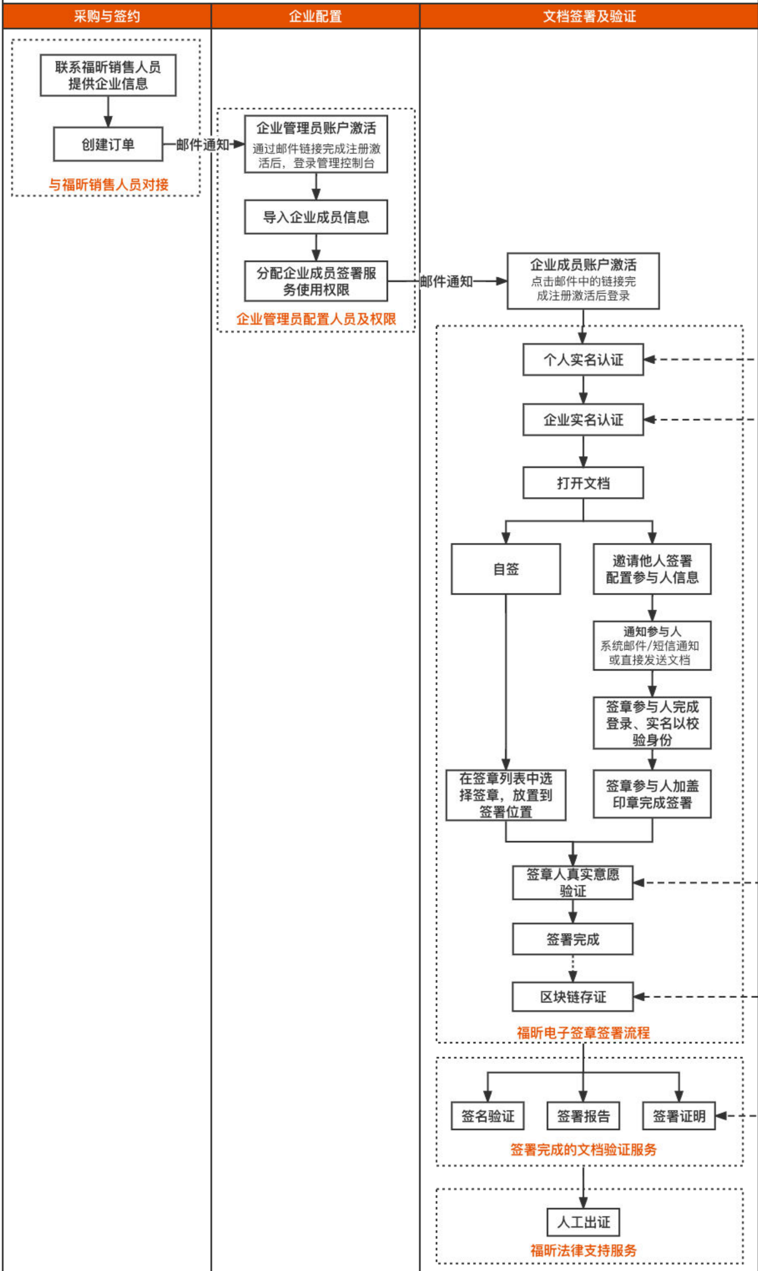
福昕电子签章服务快速使用流程简图
